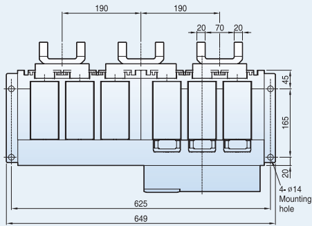
■ 3극형
