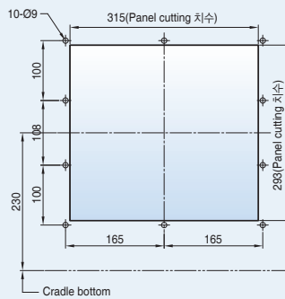
<부착구멍>
