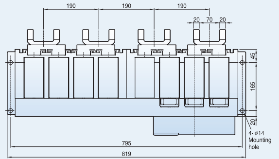
■ 4극형
