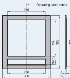
<외형크기>
