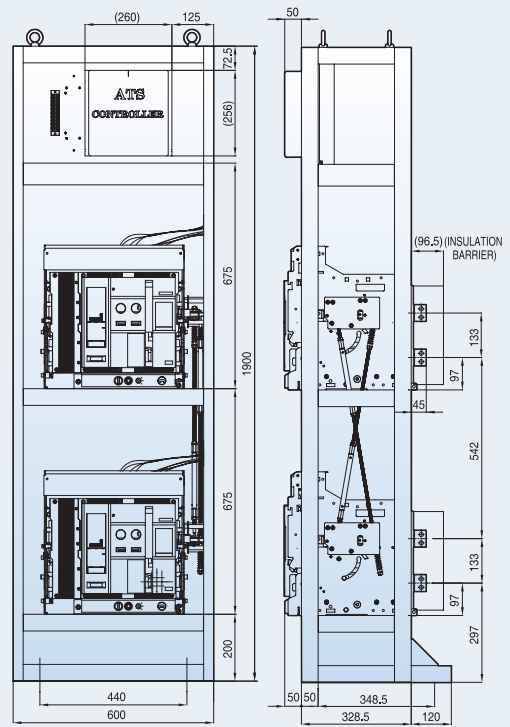
■ 16D4 (W600)
