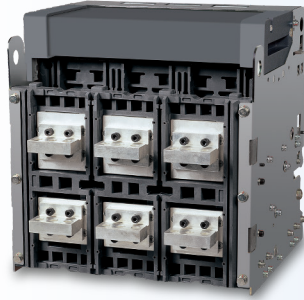
수평형 (Horizontal type)
