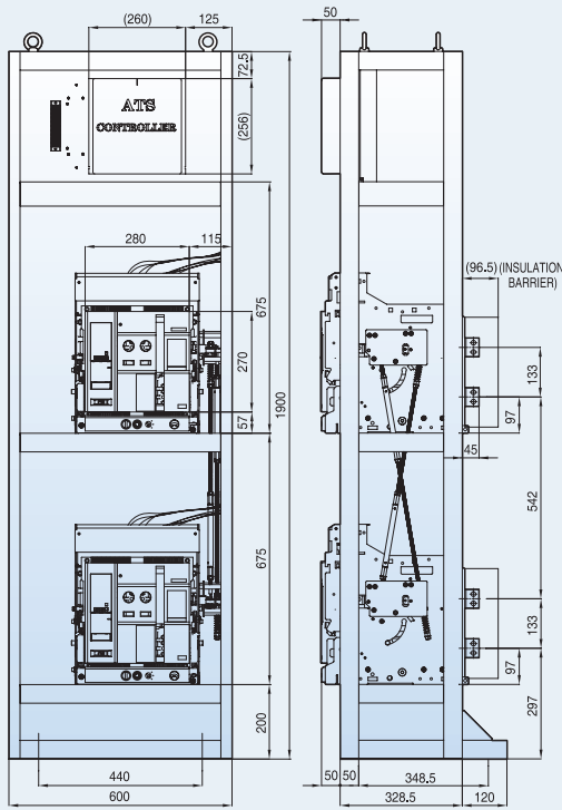
■ 16D3 (W600)
