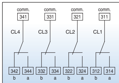
Cradle 좌측에 부착되는 4C
