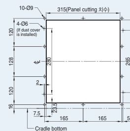
<부착구멍>
