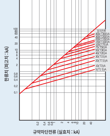
7.2kV 전류특성 M형 퓨즈 (모터보호용)
