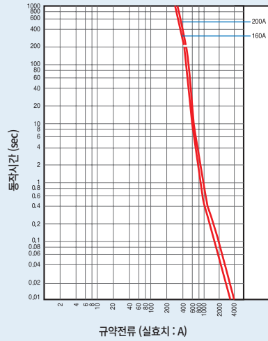
3.6/7.2kV 한류특성 M형 퓨즈 (모터보호용)
