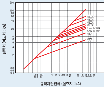
3.6/7.2kV 한류특성 M형 퓨즈 (모터보호용)
