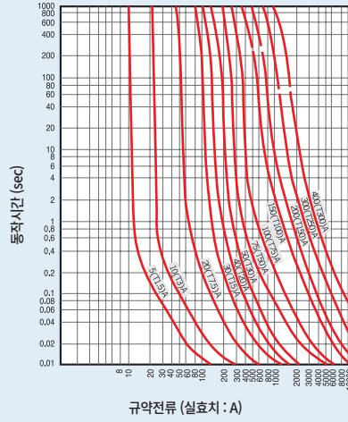
3.6kV 전류특성 M형 퓨즈 (모터보호용)
