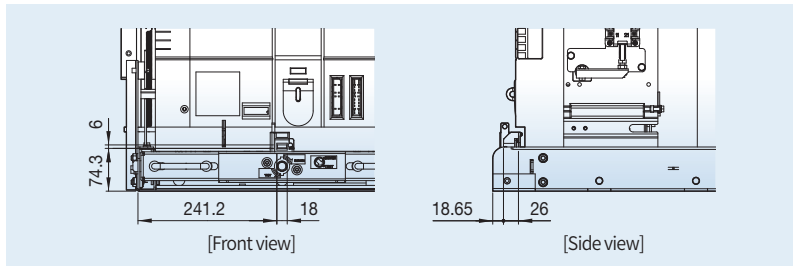
[Padlock 조립 치수(3.6/7.2kV)]
