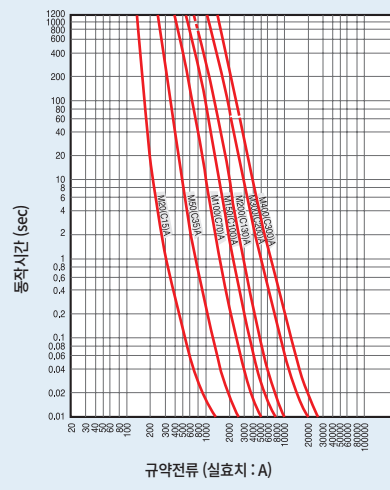
7.2kV 전류특성 M형 퓨즈 (모터보호용)
